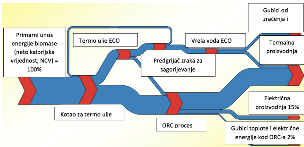
Slika 1: Energetski balans CHP postrojenja na biomasu zasnovanog na ORC tehnologiji
